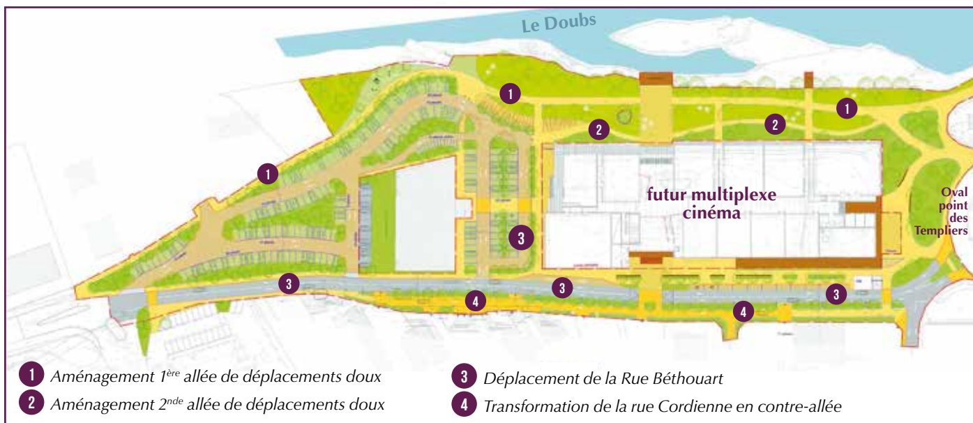
● Schéma travaux 1 ère tranche.
